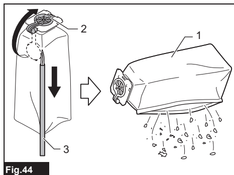
► 1. Sac à poussières 2. Capuchon de caoutchouc 3. Agrafe
